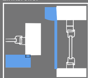
Montage auf der Fassade
