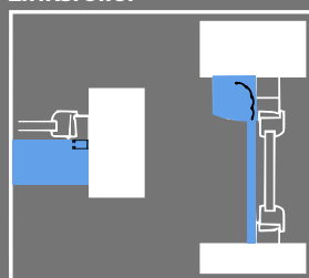
Montage in der Laibung
